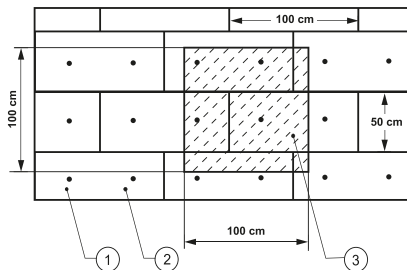
Rys.6 Schemat rozmieszczenia łączników
