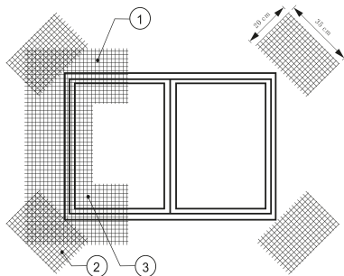
Rys.8 Montaż siatki przy otworach okiennych i drzwiowych
