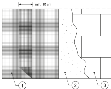
Rys.7 Montaż siatki na powierzchni ściany
