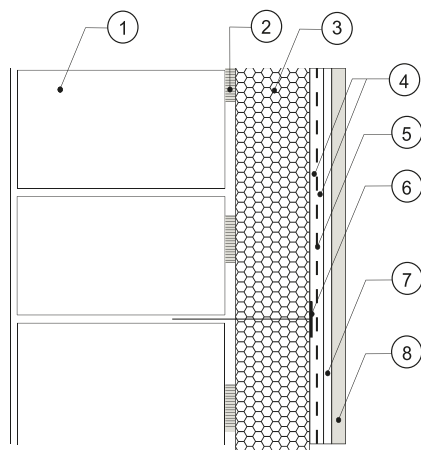
Rys.3 Warstwy ściany ocieplone w systemie ETICS
